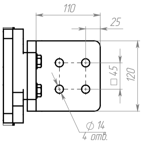
B-B (1 : 4)
